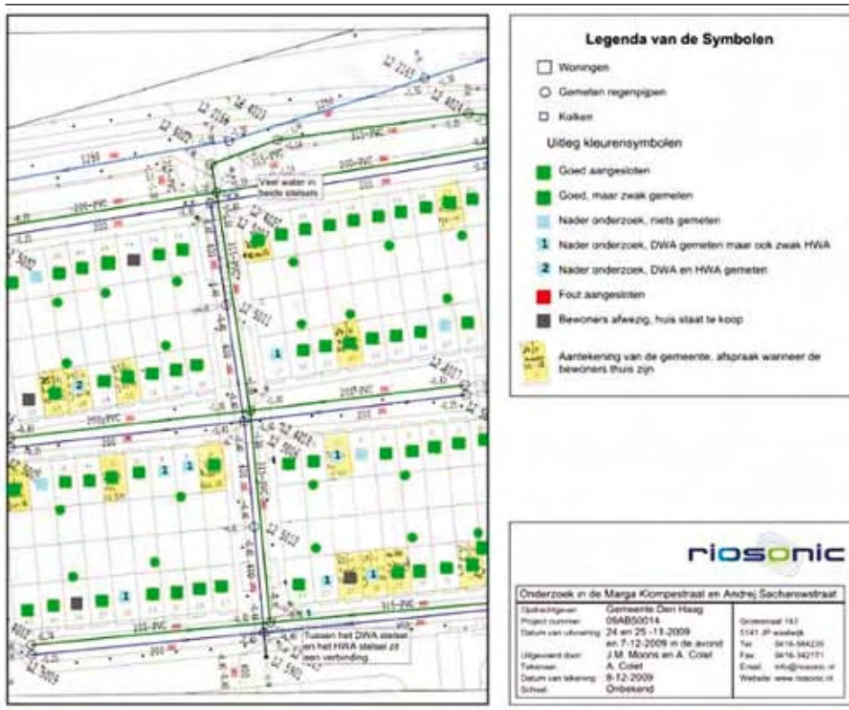
Figuur 5.12 Resultaten geluidsmeting op kleurtekening
